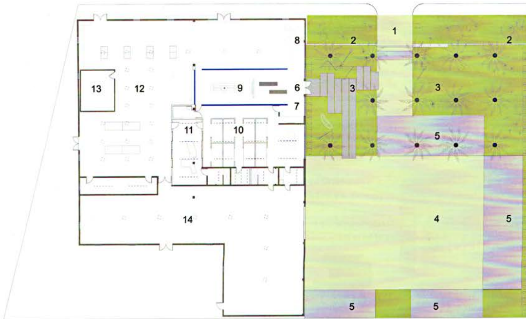
Kat planı Floor plan
